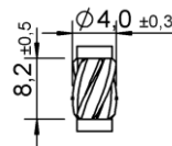
Schafffräser
