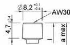
Tête cylindrique
