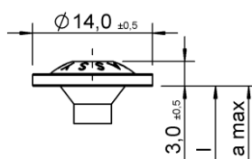
Scheiben-/Tellerkopf I
