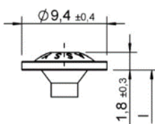
Łeb podkładowy
