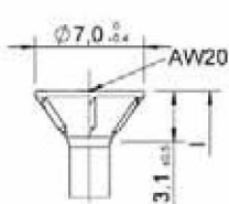
Tête fraisée à 75° avec et sans ailettes de fraissage
