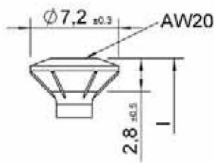
Tête FBS pour fenêtre
