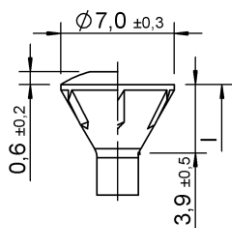
60° Holzbaukopf – mit und ohne Linse
