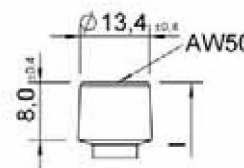
Tête cylindrique
