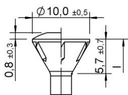
Holzbaupopf – Ausführung mit und ohne Linse
