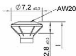
Tête FBS pour fenêtre
