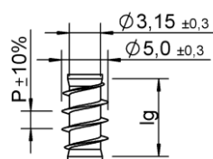
Unterkopfgewinde Lg2 < 4 x d P = 2,2; 3,1; 4,4
