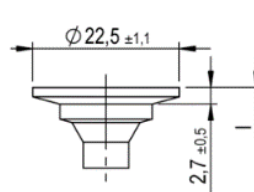
Łeb podkładkowy powiększon / talerzykowy II - z i bez krawędzi frezujących
