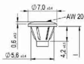
Tête Top head II - Modèle avec et sans ailettes de fraisage
