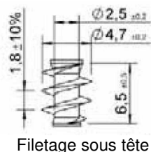
Tête Elmo
