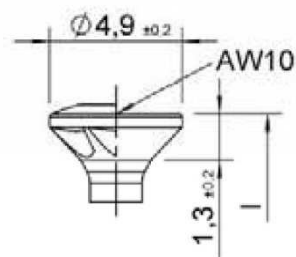
Tête pour charnière à piano : bombée ou non, avec et sans fraisoir à facettes
