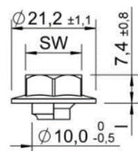
Łeb sześciokątny – z i bez wzmocnienia trzpienia / podkładki
