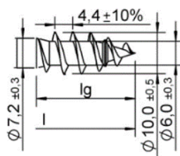
zwoj pojedynczy
