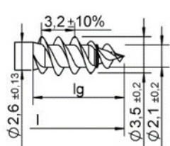
zwoj podwójny
