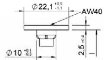
Tête à rondelle II avec et sans ailettes de fraisage
