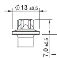
Łeb zewnętrzny Torx – z podkładką lub bez
