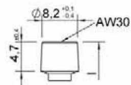
Tête cylindrique
