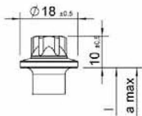
Tête hexalobulaire
