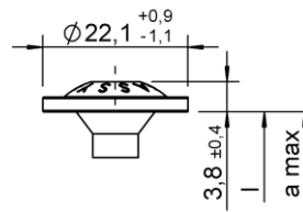
Scheiben-/Tellerkopf I
