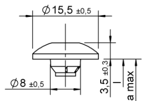
Torbandkopf – mit und ohne Fräskanten oder Schaftverstärkung
