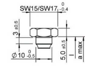
Łeb sześciokątny - zi bez wzmocnienia trzcienia / podkładki
