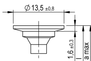
Scheiben-/Tellerkopf II
