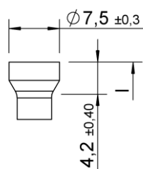
Kleiner Zylinderkopf
