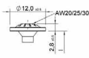
Tête à rondelle
