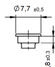
Stufenkopf
