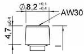
Tête cylindrique
