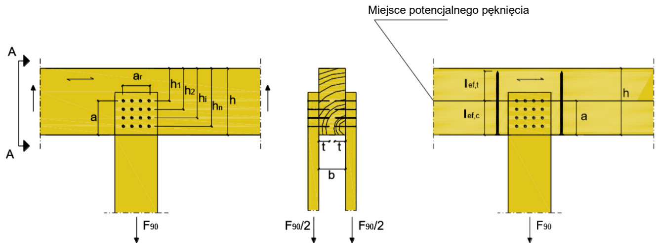
Rysunek A.4.1: Przykład wzmocnienia połączenia poprzecznego.
