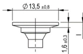
Łeb podkładowy powiększony / talerzykowy II - wersje z i bez krawędzi frezujących
