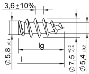
AMO Y thread
