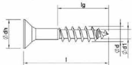
Filetage partiel sans pointe autoperceuse
