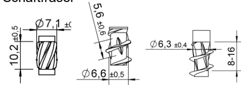
Schaftfräser
