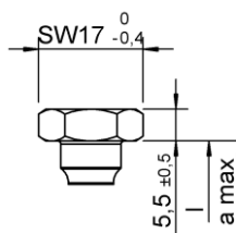
Kombikopf– mit und ohne Schaft- verstärkung/Scheibe
