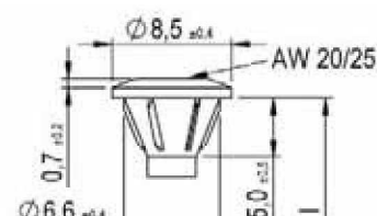
Tête Top head II - Modèle avec et sans ailettes de fraisage
