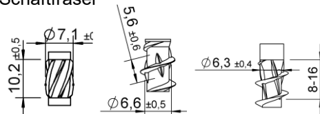
Schafffräser
