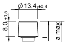
Zylinderkopf
