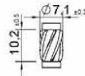
Fraisoir
