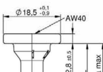
Tête à rondelle II avec et sans ailettes de fraissage
