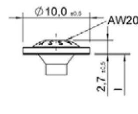
Tête pour panneau arrière
