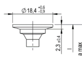
Łeb podkładowy powiększon / talerzykowy II - z i bez krawędzi frezujących
