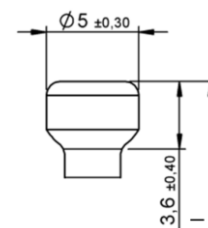
Kleiner Zylinderkopf
