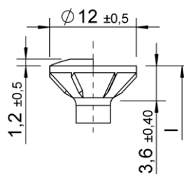
Fräskantensenkopf – mit und ohne Linse
