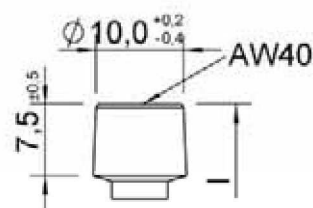
Tête cylindrique
