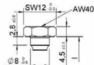
Tête Kombi
