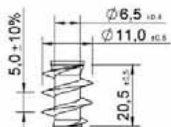
Filetage sous tête
