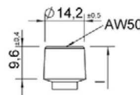
Tête cylindrique
