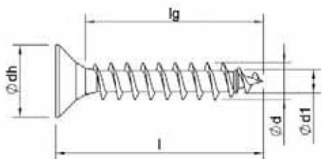
Filetage total sans pointe autoperceuse
