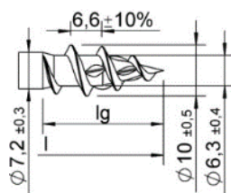
grubozwojny II
