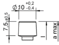
Łeb walcowy
