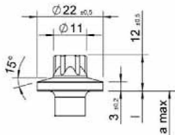
Tête hexalobulaire
