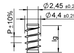
Unterkopfgewinde Lg2 < 4 x d, P = 1,8; 2,2
