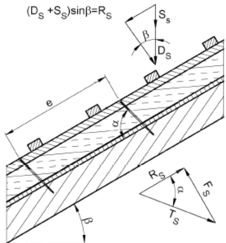
Figure 5.3 : Charges isolées F_s perpendiculaires aux contre-lattes, application des charges au niveau de la tête des vis
