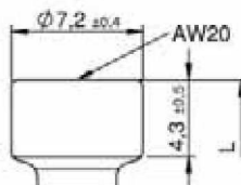
Tête cylindrique
