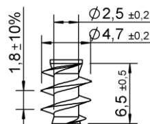
Unterkopfgewinde Typ P
