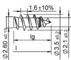
zwoj pojedynczy
