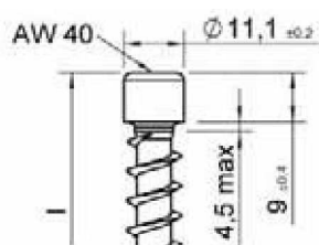
Tête cylindrique
