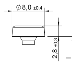
Elmo Kopf
