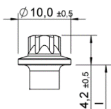
Łeb zewnętrzny Torx – z podkładką lub bez
