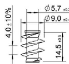
Filetage sous tête
