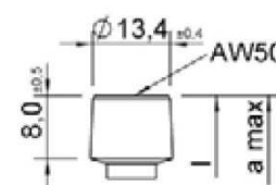
Tête cylindrique
