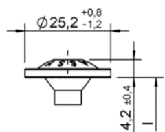
Łeb podkładkowy powiększon / talerzykowy I
