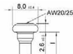
Tête de vis pour sabot
